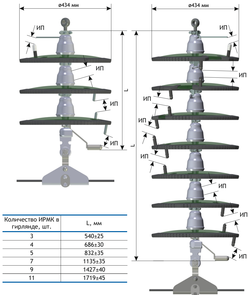
Рисунок 10 - Эскиз установки, а также габаритные, установочные и присоединительные размеры
